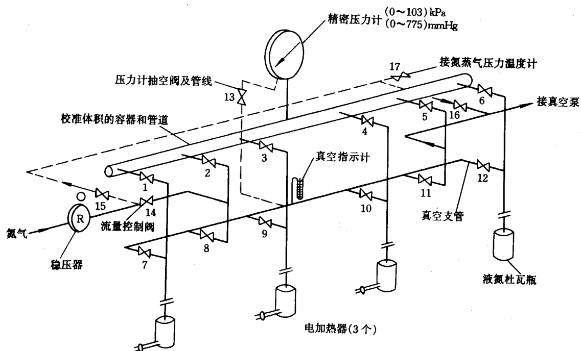
图1 四试样管 Ni-Count-1 比表面积测定仪简图
