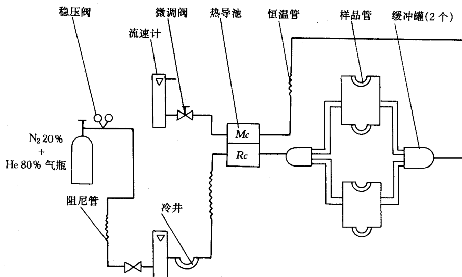
图 4 高效动态吸附仪图
