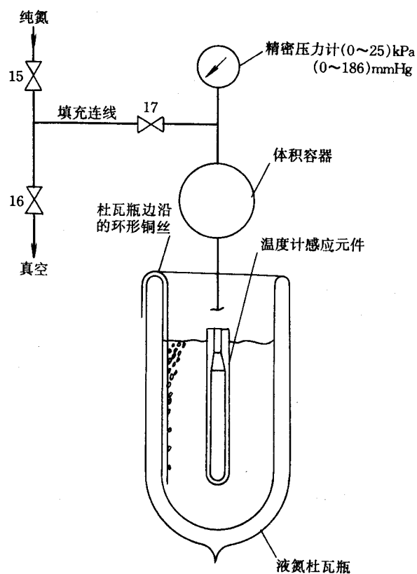
图2 氮蒸气压力温度计
