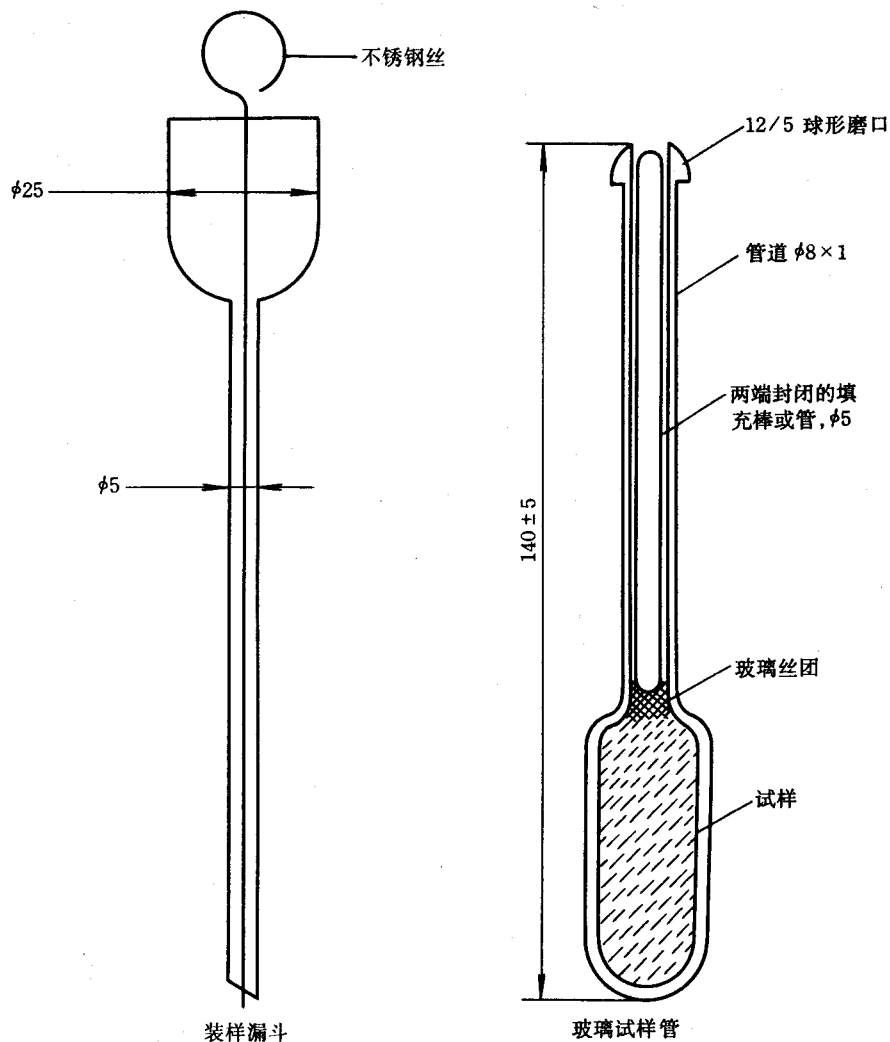
图 3 装样漏斗及玻璃试样管
